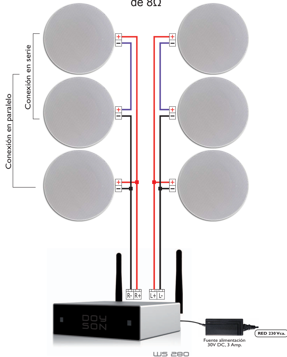
Instalación con 6 Altavoces de 8Ω
