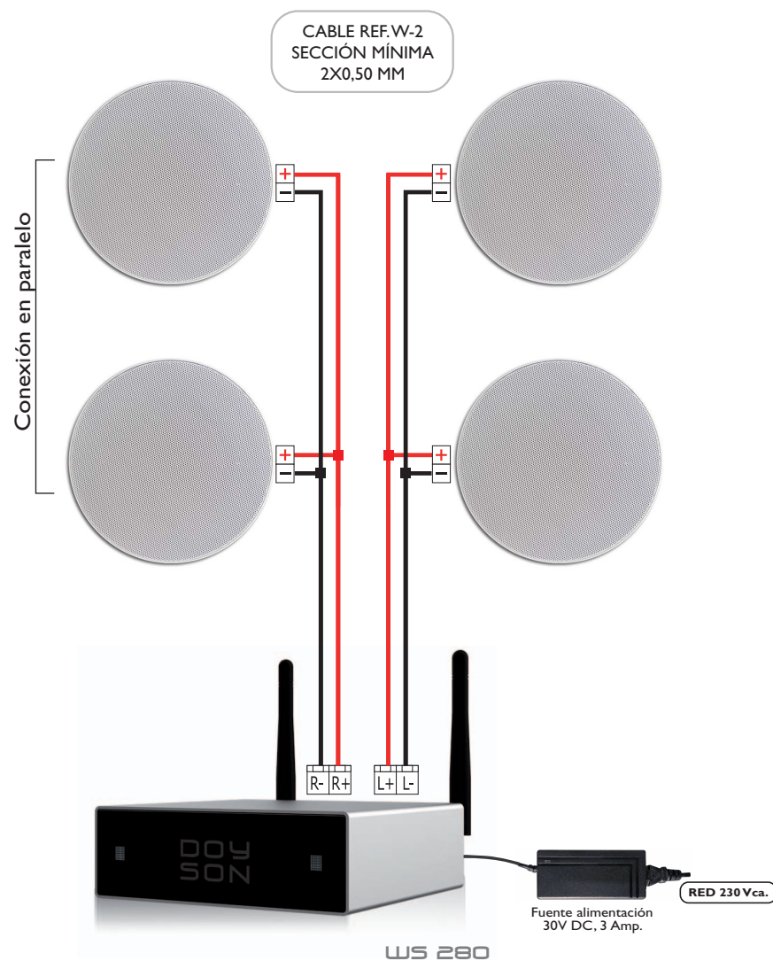
Instalación con 4 Altavoces de 8Ω
