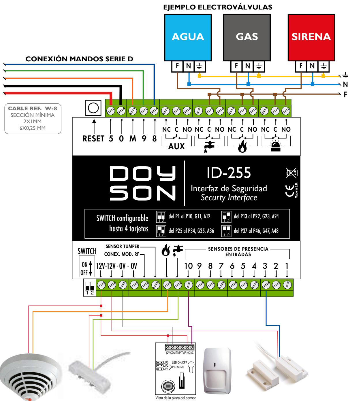
EJEMPLO DE CONEXIÓN DE SENSORES
